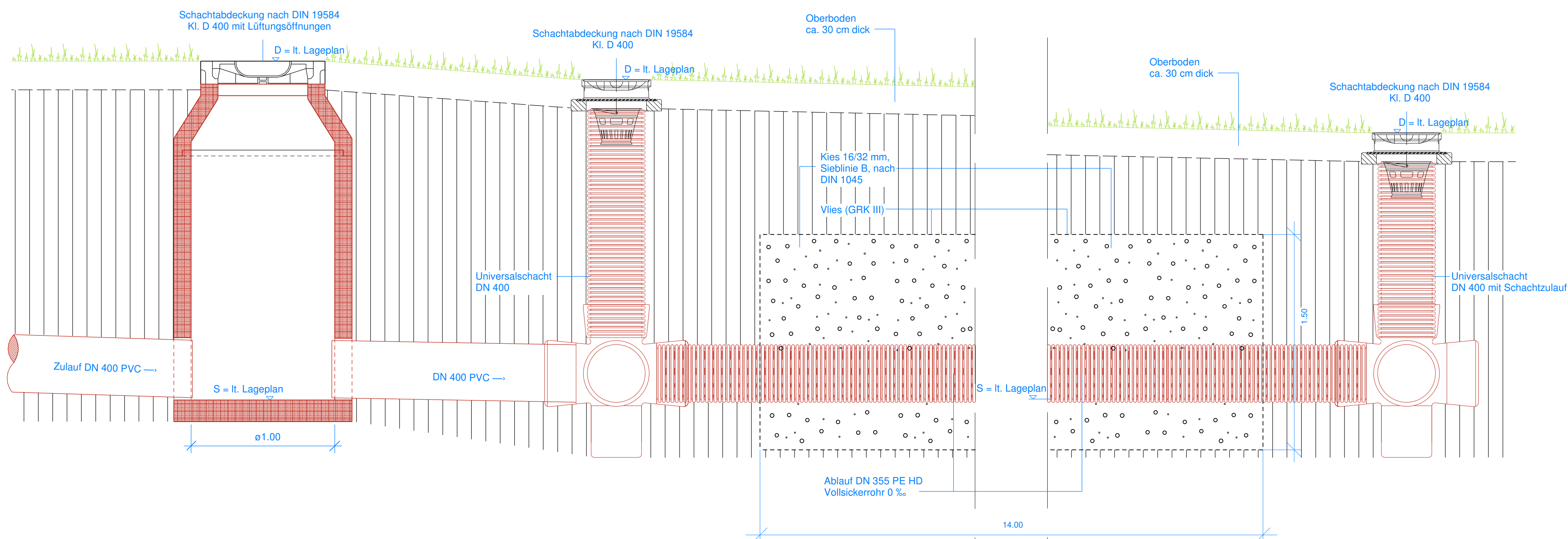
Schnitt A-A
